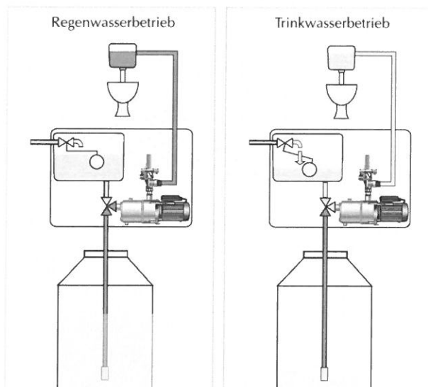
Bild 2 Regenwasser- und Trinkwasserbetrieb
