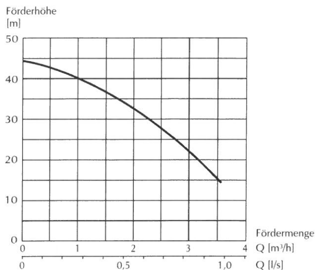
Bild 5 Pumpenkennlinie: Fördermenge in Abhängigkeit von der Förderhöhe
