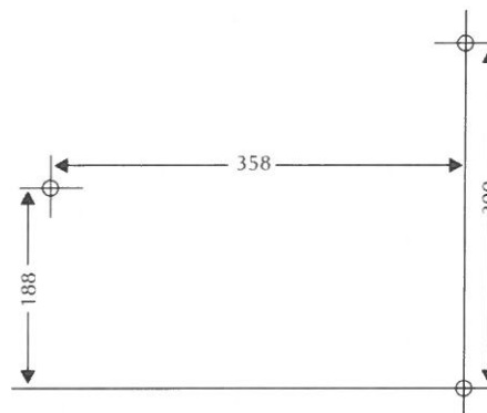
Bild 7 Lochschablone für Wandmontage Box V50E
