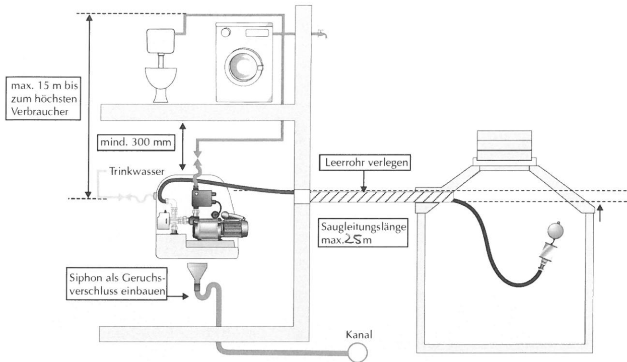
Bild 8 Hydraulischer Anschluss der Box V50E
