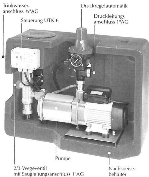
Bild 4 Aufbau
