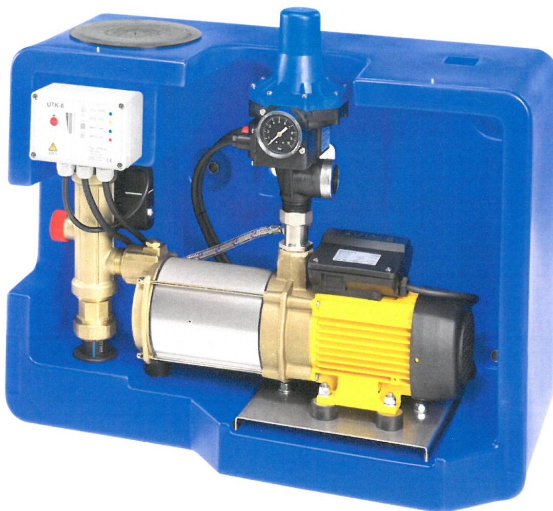
Bild 1 Box Komfort V
