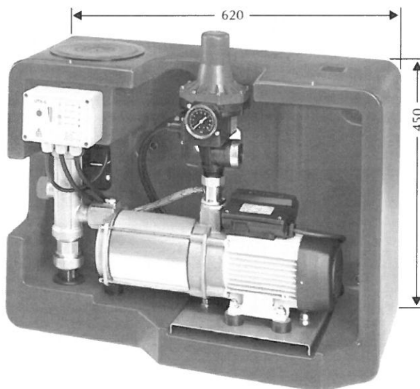
Bild 6 Maße und Anschlüsse
