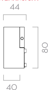
K200 IMPULSGEBER, SEITENANSICHT
