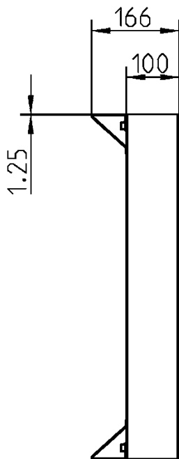
Fußgestell DWT 750 l + 1000 l Werkstoff: DX 51 D Z275 alternativ: DX 51 D ZA255
