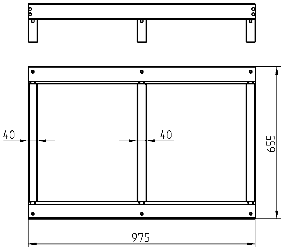
Fußgestell DWT 750 l + 1000 l Werkstoff: DX 51 D Z275 alternativ: DX 51 D ZA255
