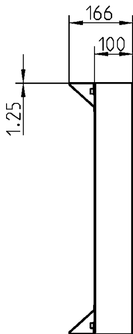
Fußgestell DWT 620 l Werkstoff: DX 51 D Z275 alternativ: DX 51 D ZA255
