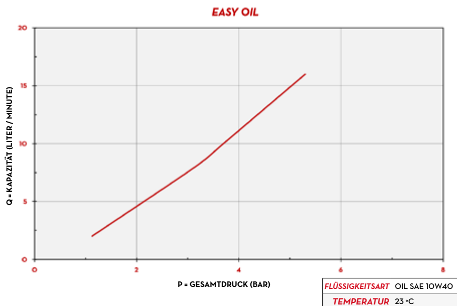
1/2" EINGANG
