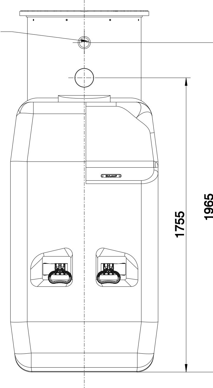
Seitenansicht: Zulauf
