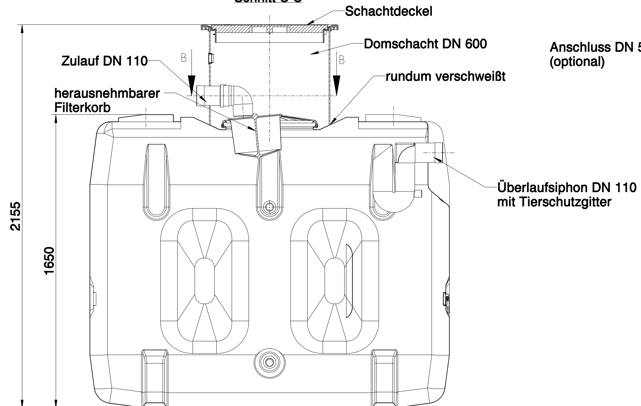
Schnitt C-C
