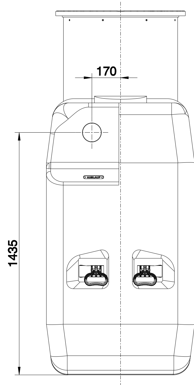
Seitenansicht: Überlauf
