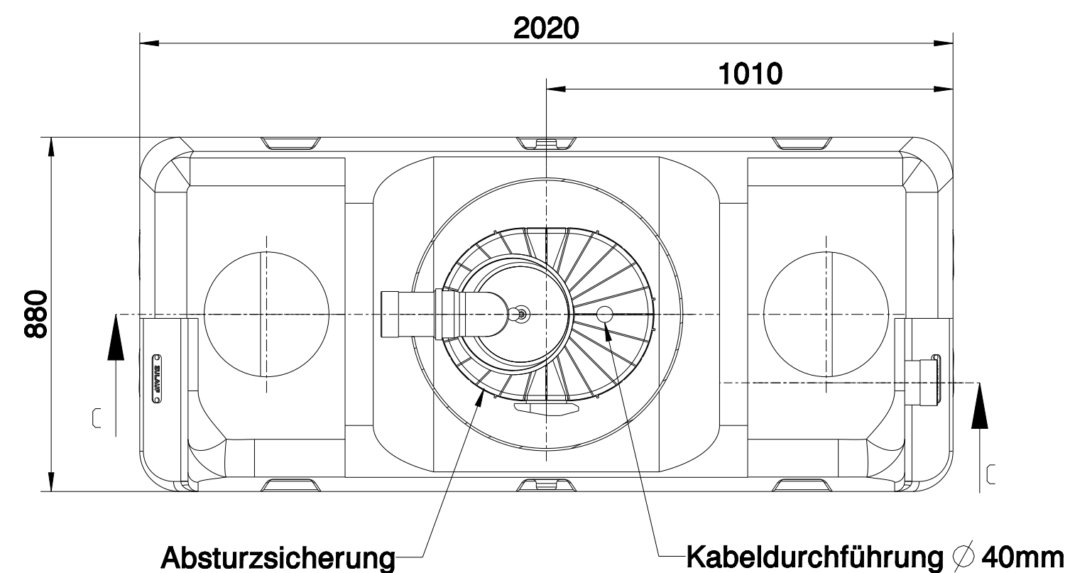
Schnitt B-B
